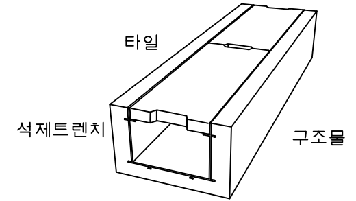
설치예시도 scale : None
