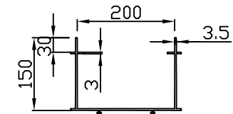
정면도 scale : None
