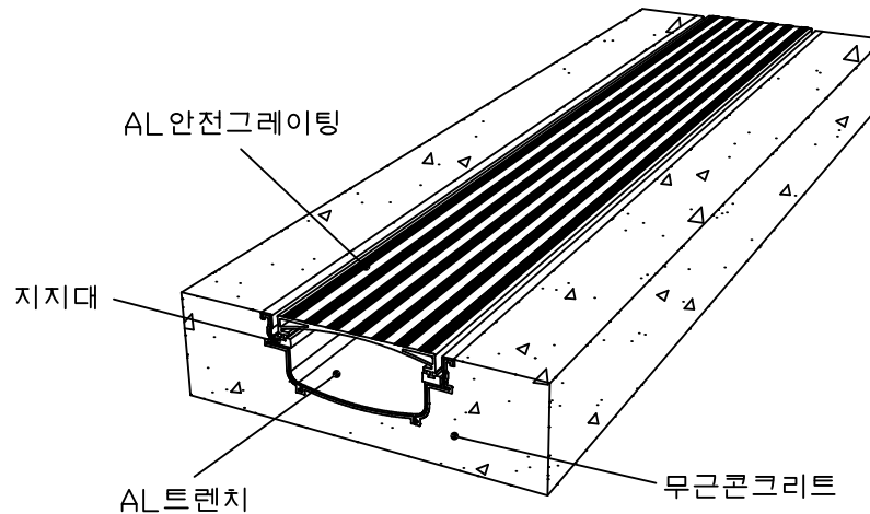
설치예시도 scale : None
