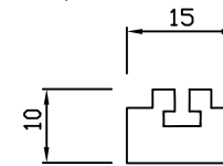
정 면 도 scale : None
