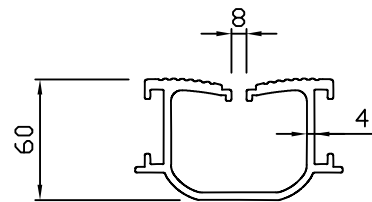
정면도 scale : None
